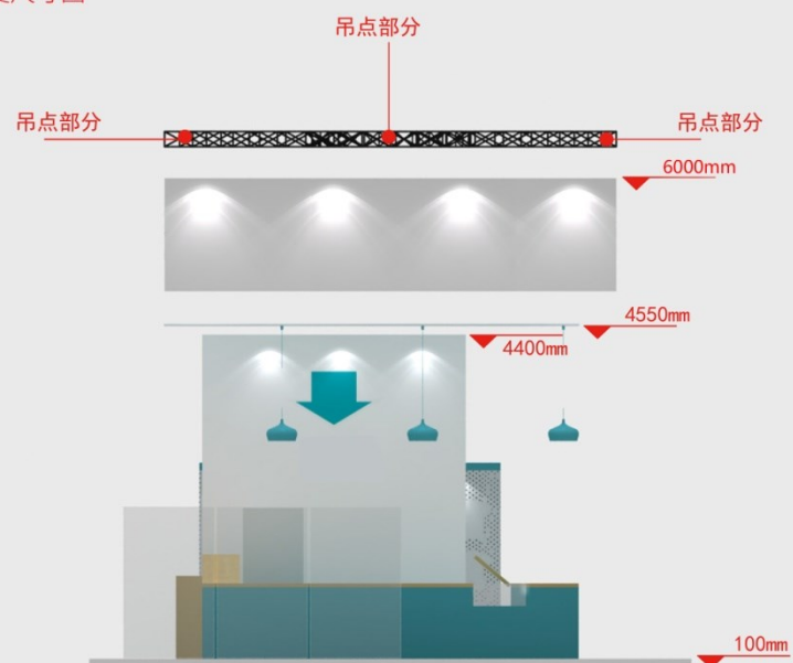
4.吊挂物离地高度尺寸图
